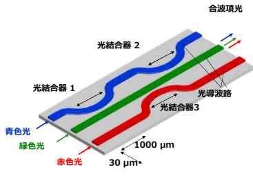
光導波路型合波器の構造
